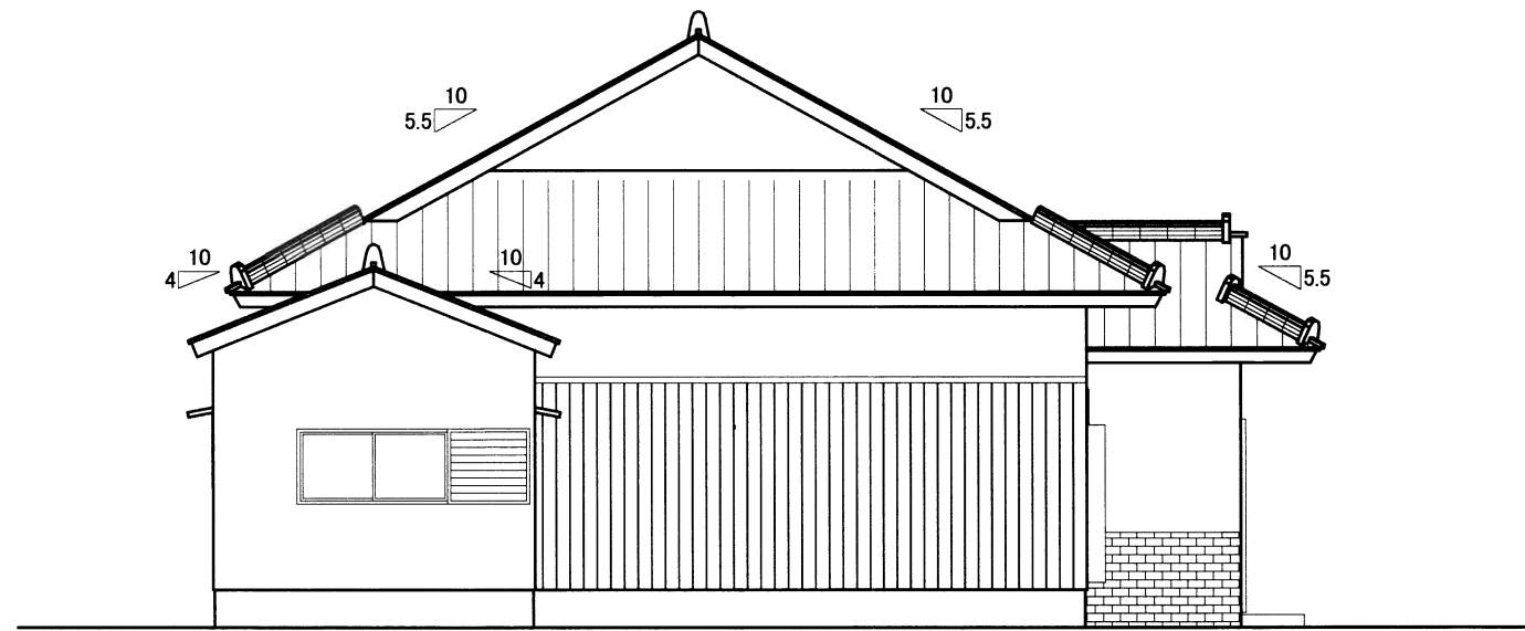
西側立面図
