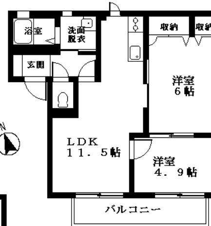
C 間取図 反転タイプ有り
